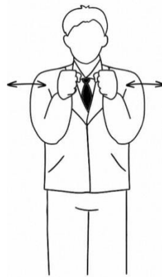
Odpychanie
